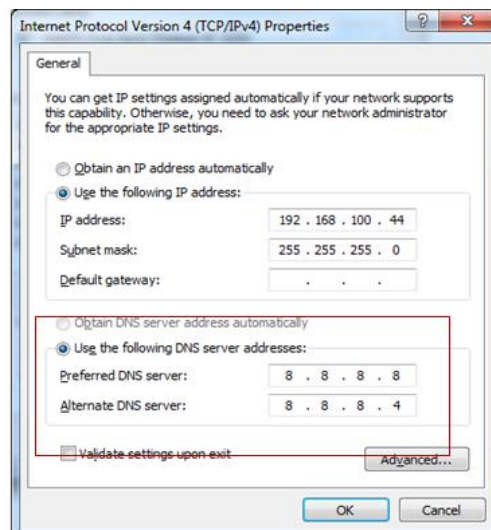
(Dialog box 5)
