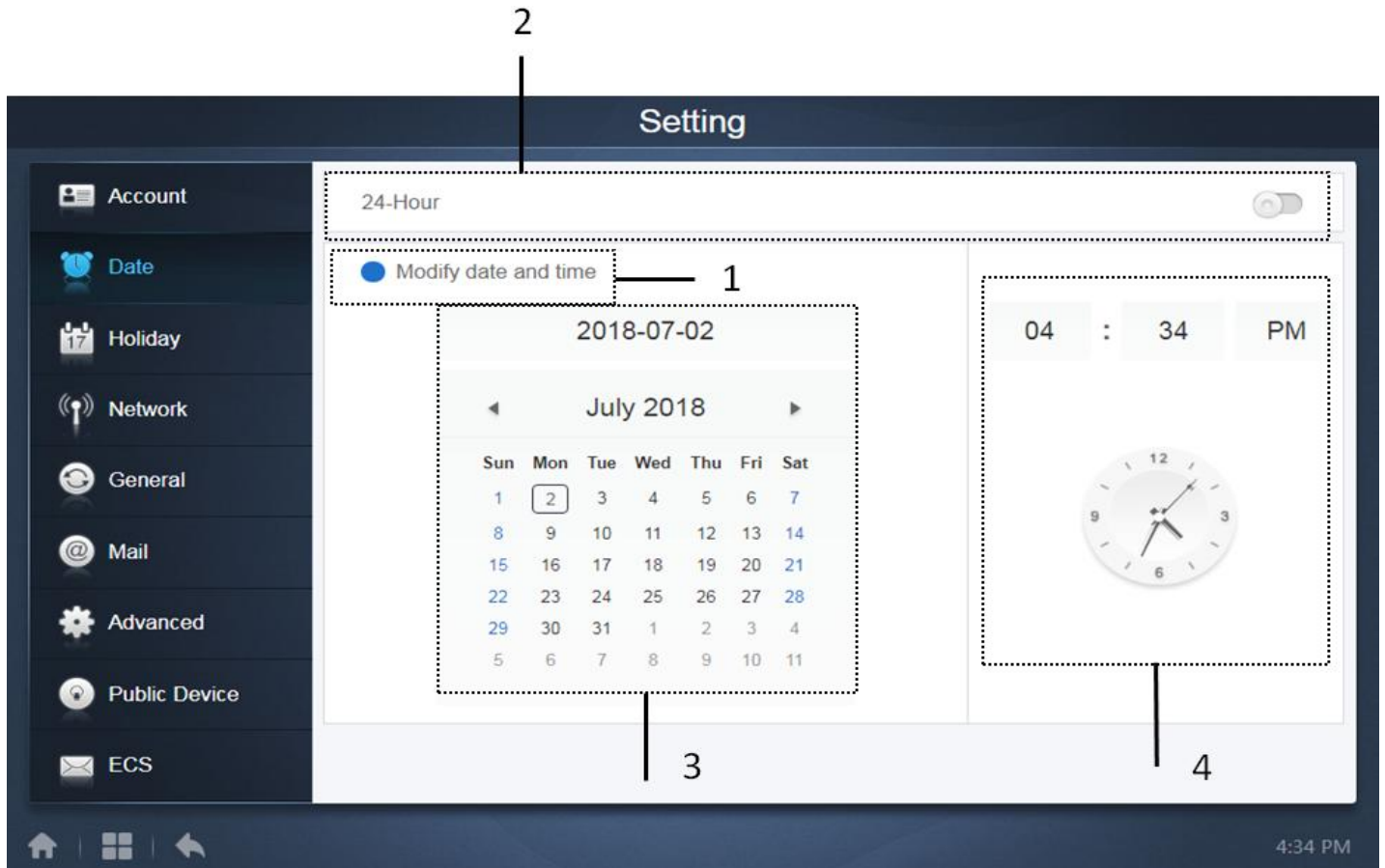
(Default display)
